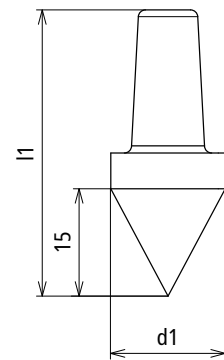
Maßbild
