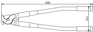
Maßbild HVI CUTTER 32
