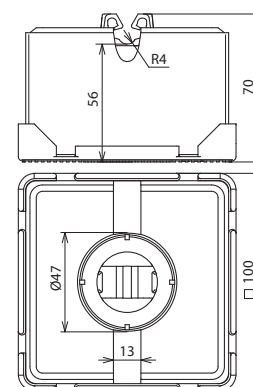
Maßbild DLH FB 8 LO 100X100X70
