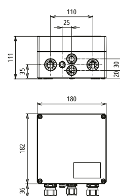
Maßbild DCU 2 YPV 1+2 1000 1M 2S FM
