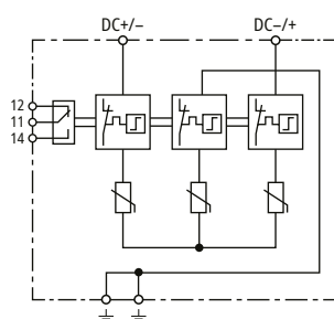
Prinzipialschaltbild DCU 2 YPV 1+2 1000 1M
