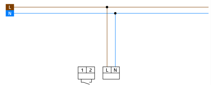
Schaltbild
