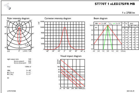
IFAS1_ST770T1xLED27SFRMB
