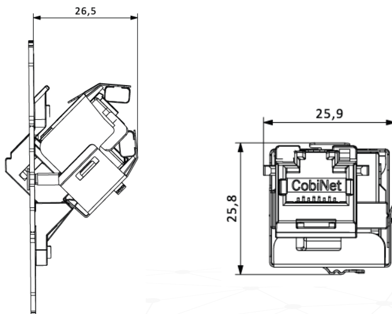
Abb.1: RJ45-TL® rapid in Anschlussdose (Art.-Nr.: 127138)
