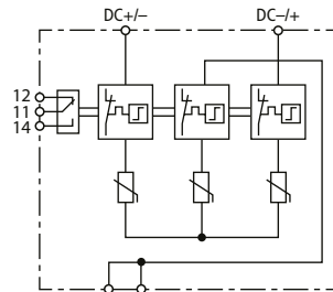
Prinzipschaltbild
