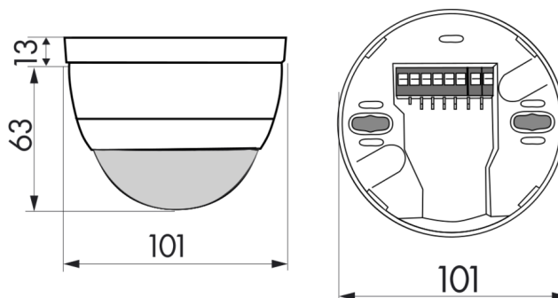
Bemaßung 92440
