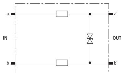
Prinzipschaltbild DRL RD 12
