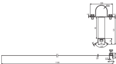
Maßbild BS D50 DS90 SB50.300 V2A
