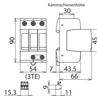
Maßbild DG M TNC 275 FM
