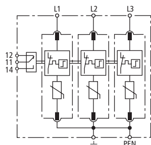
Prinzipschaltbild DG M TNC 275 FM
