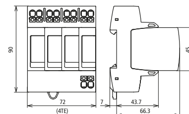
Maßbild DG MP TNS 275
