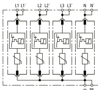
Prinzipschaltbild DG MP TNS 275
