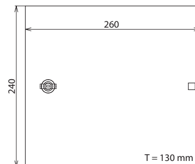
Maßbild DPG LSA 30 P
