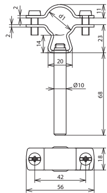
Maßbild LH ZS 20 23 DS10 L75 V2A
