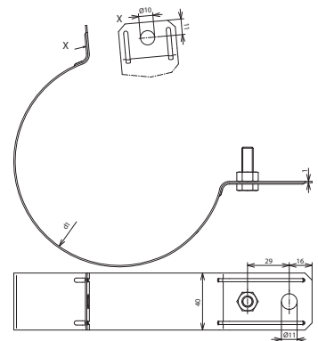
Maßbild RRS 100 B11 CU
