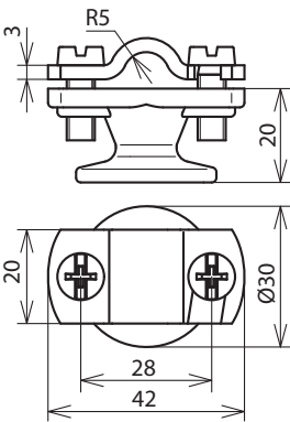
Maßbild LH ZS 7.10 IGM8 STTZN ZG
