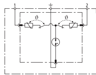
Prinzipschaltbild DR M 2P 255 SN1802
