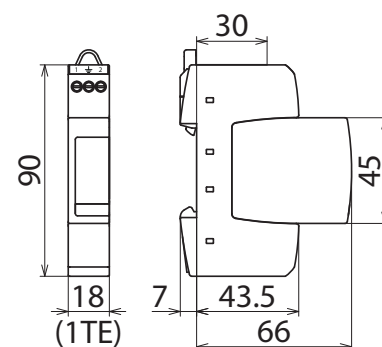
Maßbild DR M 2P 255 SN1802
