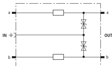
Prinzipschaltbild DRL RE 48
