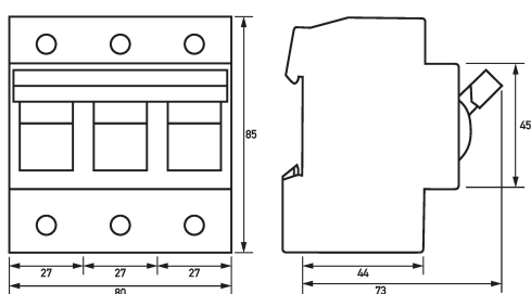
Maßzeichnung Sicherungslasttrennschalter Coron 2 Do-63-3
