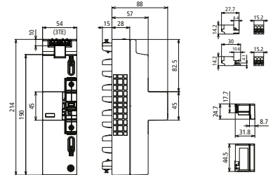
Maßbild DSH ZP B2 LSG A TT 255
