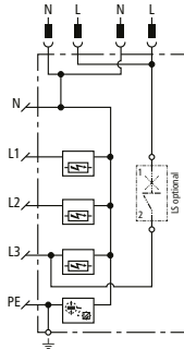
Prinzipialschaltbild DSH ZP B2 LSG A TT 255
