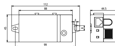
Maßbild DBX TC B 180
