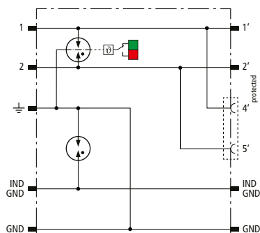
Prinzipschaltbild DBX TC B 180
