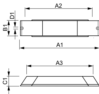
HID-PV m 20 // CDM HPF 220-240V 50/60Hz
