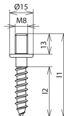
Maßbild HSC 8X32 AGM8X13 STGALZN
