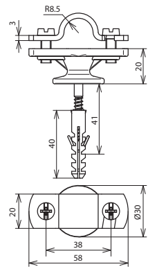
Maßbild SH ZS 16 KD8X40 STTZN ZG
