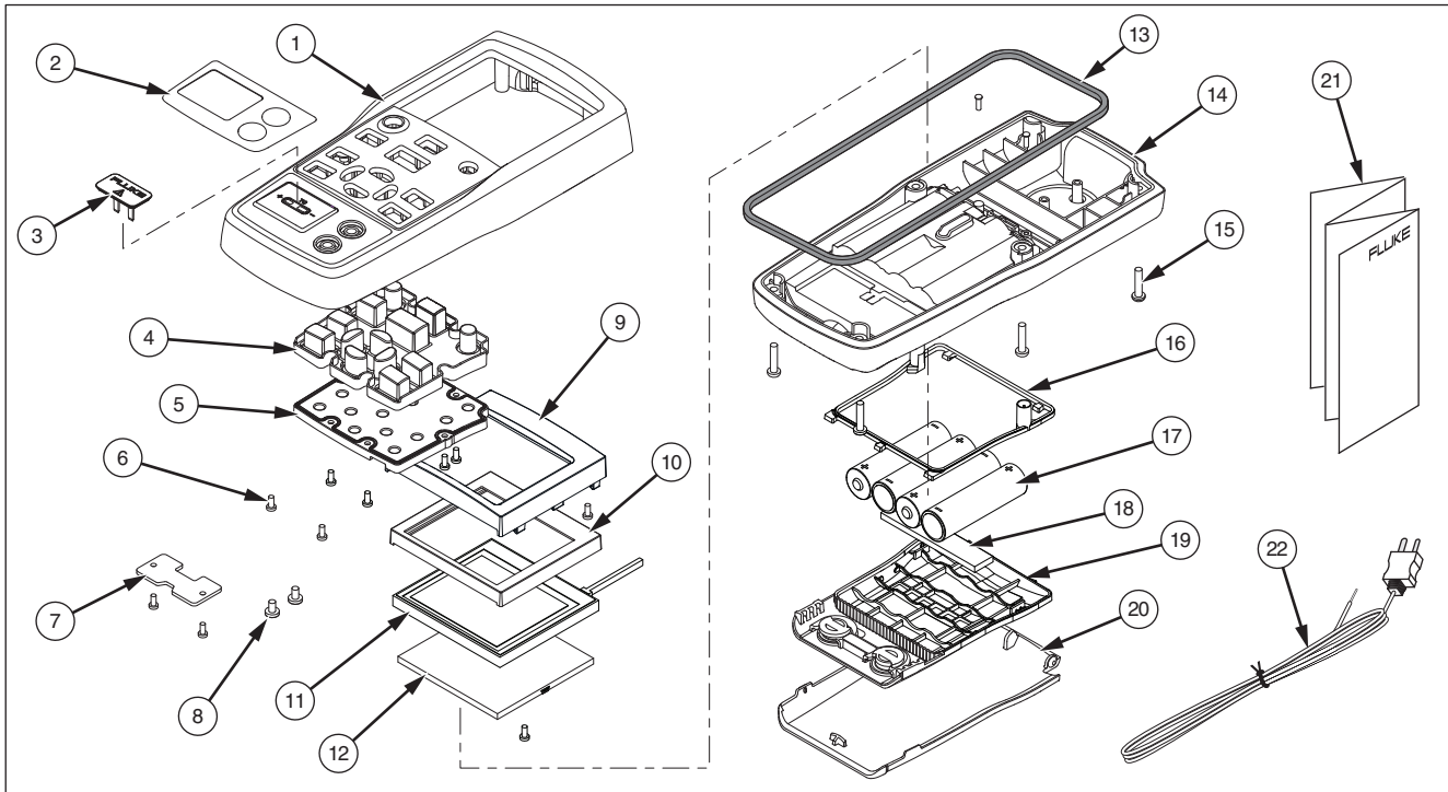
Abbildung 9. Ersatzteile
