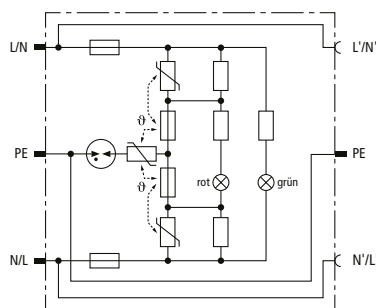
Prinzipschaltbild DPRO 230
