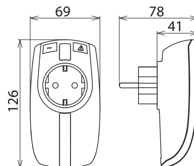
Maßbild DPRO 230
