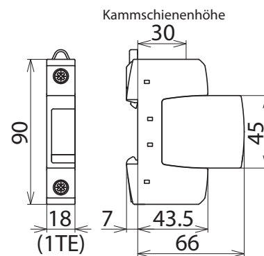
Maßbild DG S 275
