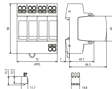
Maßbild DG MP TNS 275 FM
