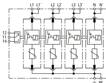
Prinzipialschaltbild DG MP TNS 275 FM
