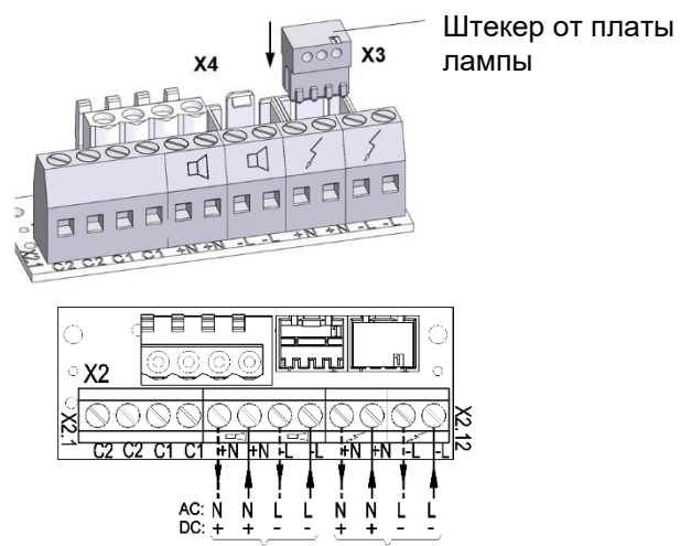
Подключение рабочего напряжения излучателя звука
