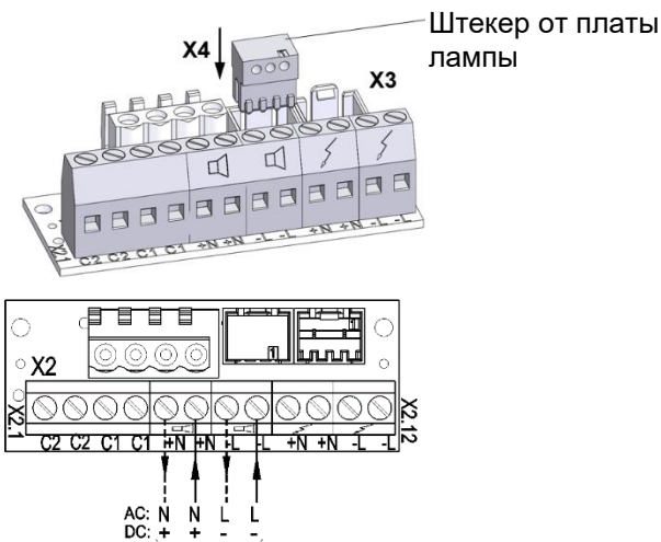
Подключение рабочего напряжения
