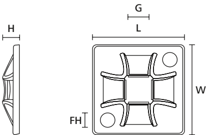
Q-Mount (Seitenansicht)
