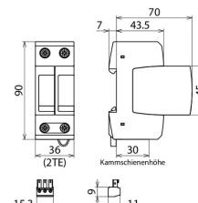
Maßbild DG M TT 2P ACI 275 FM
