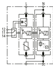
Prinzipialschaltbild DG M TT 2P ACI 275 FM
