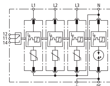
Prinzipschaltbild DG M TT 275 FM
