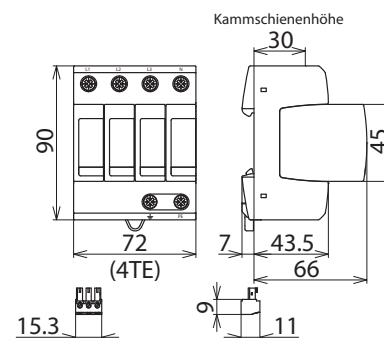
Maßbild DG M TT 275 FM
