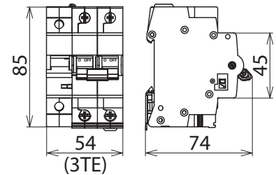
Maßbild POP 2 255 C32
