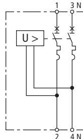
Prinzipschaltbild POP 2 255 C32
