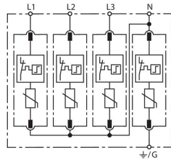
Prinzipialschaltbild DG MU 3PY 480 4W+G
