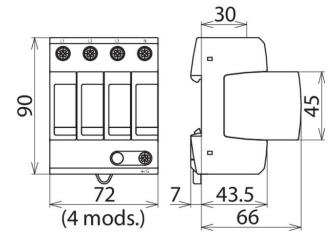
Maßbild DG MU 3PY 480 4W+G
