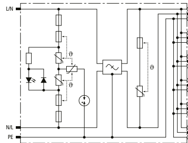
Prinzipschaltbild
