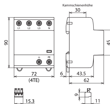
Maßbild DSH TNS 255 FM
