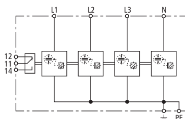
Prinzipschaltbild DSH TNS 255 FM
