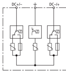
Prinzipialschaltbild DG YPV SCI 600
