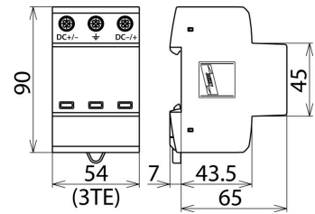
Maßbild DG YPV SCI 600
