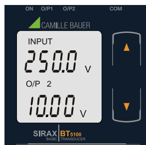
Anzeige 5: Spannungs- Eingang und Ausgang 2 als Spannung
