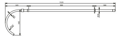
Maßbild RST 72.5 1500
