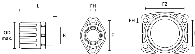
HeliaGuard Verschraubung, gerade drehender Flansch
