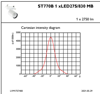
IFCC1_ST770B1xLED27S830MB
