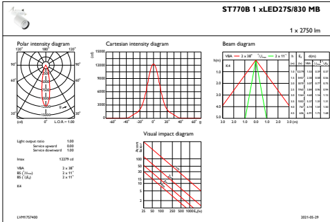
IFAS1_ST770B1xLED27S830MB
