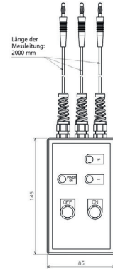
Maßbild
