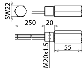
Maßbild DPI CD EXD 24 M
