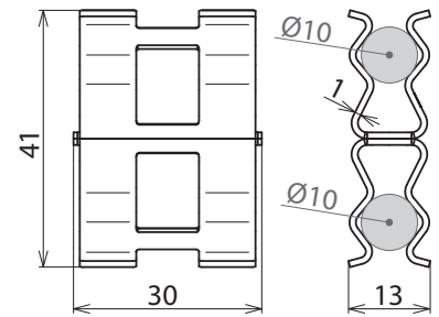
Maßbild DC BK 10 RD10 STBLANK
