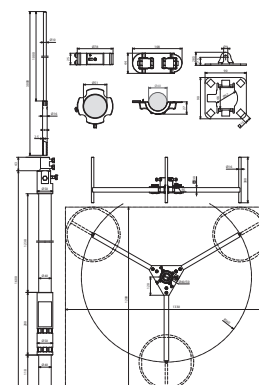
Maßbild FM D40 L4700 GFK AL DBS R560
