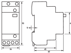
Maßzeichnung Gruppenansicht
