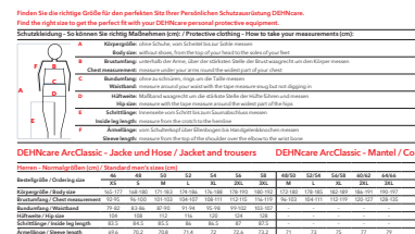
Maßbild APT 50
