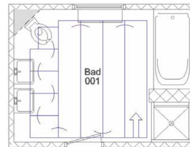
DEVI Verlegeplan
