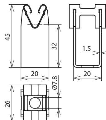
Maßbild LH DG 8 H32 B7.8 V2A
